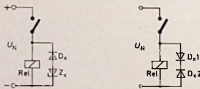
Bild 10. Spannungsbegrenzung mit gegen geschalteten Null-Dioden
