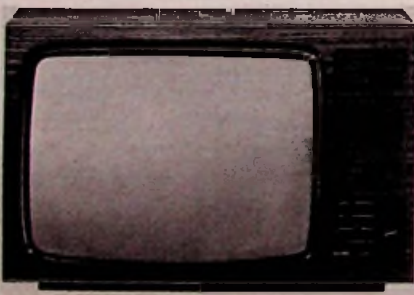
Marke: Graetz Modellname: Kornett color electronic 2647 Erstlieferung a. d. Handel: April 1975 Unverbindliche Preisempfehlung: 2109/2149 DM Bilddiagonale: 66 cm Fernbedienung: nein Gehäuseausführung: Dekor Nußbaum oder Altweiß
