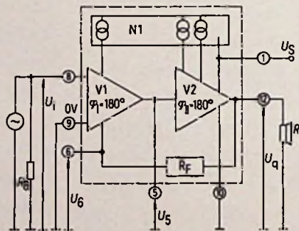
Bild 1. Blockschalbild des NF-Leistungsverstärkers TBA 810
