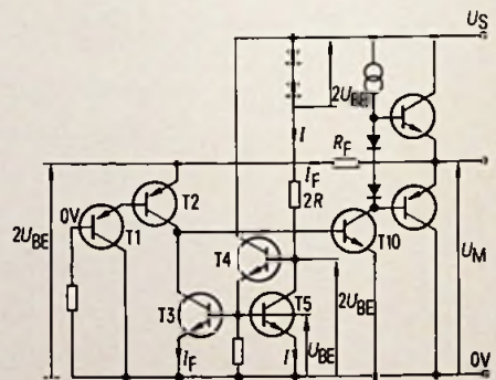
Bild 3. Erweitertes Prinzipschalbild des Leistungsverstärkers
