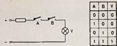
Bild 4. Symbolische Darstellung einer UND-Schaltung und Wahrheitstabelle
