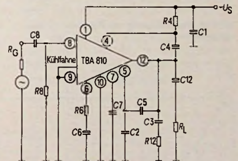
Bild 9. Beschaltungsmöglichkeiten der IS. R_4 = 100 \Omega , R_6 = (siehe Text), R_8 = 100 \text{ k}\Omega , R_{12} = 1 \Omega , R_L = 4 \Omega , C_1 = 100 \text{ nF} , C_2 = 2,7 \text{ nF} , C_3 = 100 \text{ nF} , C_4 = 100 \mu\text{F} , C_5 = 560 \text{ pF} , C_6 = (siehe Text), C_7 = 100 \mu\text{F} , C_8 = 100 \text{ nF} , C_{12} = 1000 \mu\text{F}
