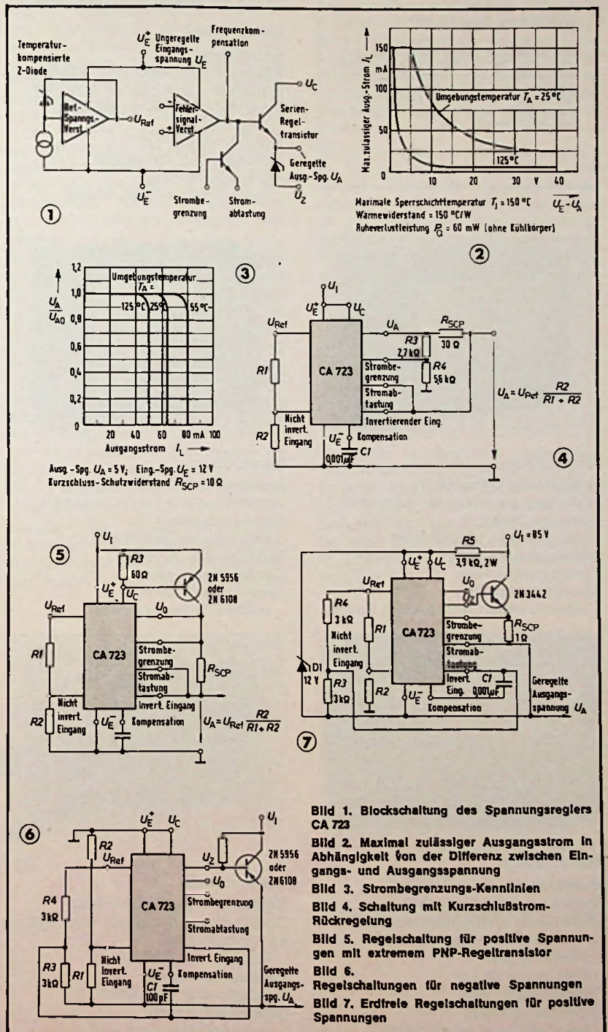
Bild 7. Erdfreie Regelschaltungen für positive Spannungen
