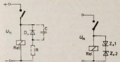
Bild 5. Störspannungsbegrenzung mit Null-Diode D_x und RC-Kombination
