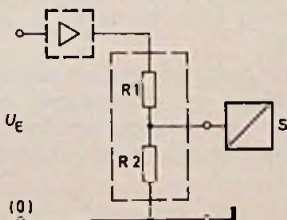
Bild 13. Störspannungsschutz mit Spannungsteiler R_1 , R_2
