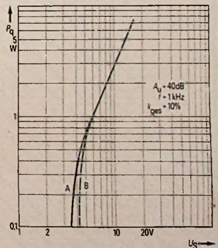
Bild 10. Ausgangsleistung als Funktion der Betriebsspannung
