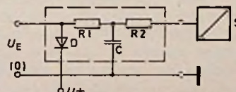
Bild 16. Störspannungsschutz mit Begrenzungsdiode D und Integrierglied
