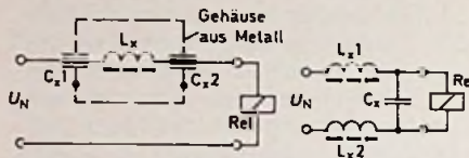
Bild 7. Einleiterentstörung mit Durchführkondensatoren C_{x1} , C_{x2}
