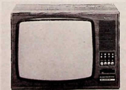
Marke: Siemens Modellname: Bildmeister FC 503 superelectronic Erstlieferung a. d. Handel: Mai 1975 Endverkaufspreis: liegt bei etwa 1950 DM Bilddiagonale: 56 cm Fernbedienung: nein Gehäuseausführung: Nußbaum-Dekor hell
