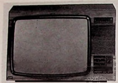
Marke: Graetz Modellname: Reichsgraf color electronic 2648 H Erstlieferung a. d. Handel: April 1975 Unverbindliche Preisempfehlung: 2158/2198 DM Bilddiagonale: 66 cm Fernbedienung: Ultraschall Gehäuseausführung: Dekor Nußbaum oder Altweiß
