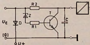
Bild 17. Aktive Störspannungs-Kurzschluß-Schaltung
