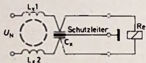
Bild 9. Zweileiterentstörung mit Ringkerndrossel und Y-Kondensator
