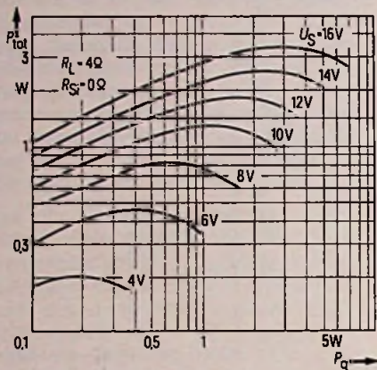
Bild 12. Verlustleistung als Funktion der Ausgangsleistung
