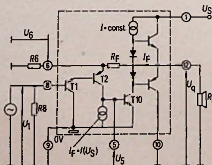
Bild 2. Prinzipschalbild des Leistungsverstärkers
